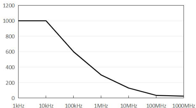
最大有效值 (Vrms) VS 频率曲线
