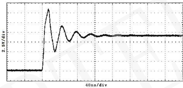
添加输入延长线的波形
