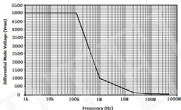
图 4 DPR6700A 最大差模电压 VS 频率
