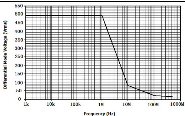
图 1 DPR6070A 最大差模电压 VS 频率
