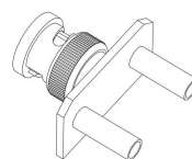
图二 BNC 公头转双香蕉头母头
