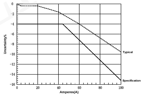
图 4 典型的 DC 线性度 (0.01V/A 档位)
